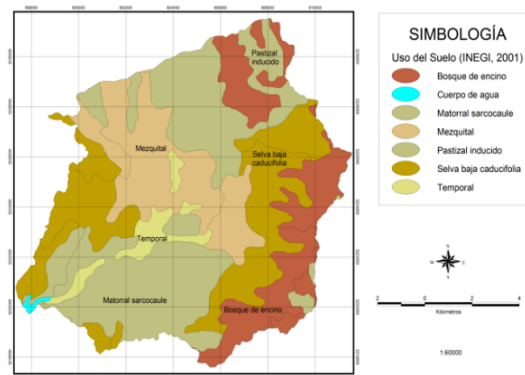
Figura 47. Tipos de Vegetación según INEGI (1981a; 2006a).
