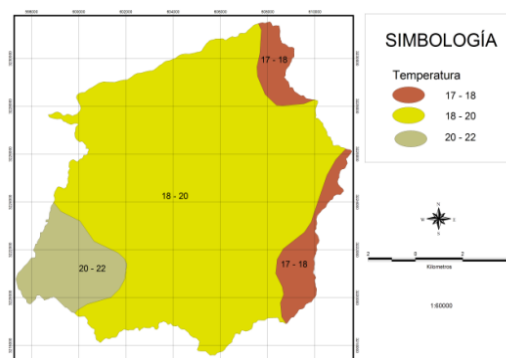
Figura 23. Isotermas (INEGI, 1985).
