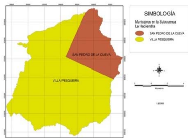
Figura 7. Municipios en la Subcuenca La Haciendita.
