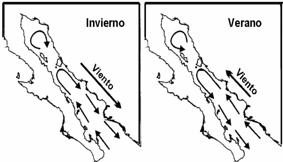
Figura 5. Modelo de circulación superficial del mar en el Golfo de California durante invierno y verano (tomado de Lluch-Cota 2000).
